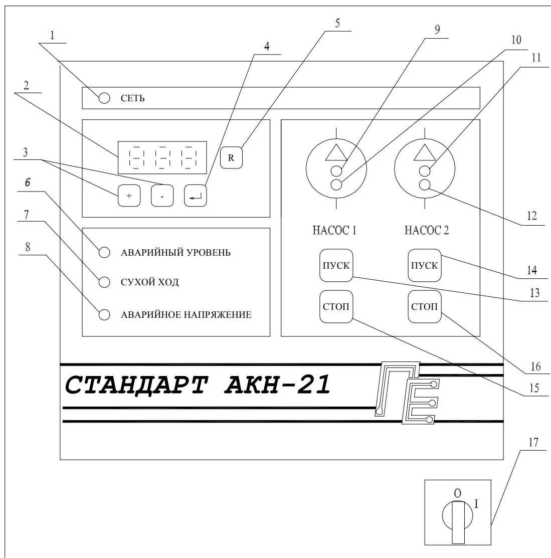
Рисунок 1 – Лицевая панель устройства СТАНДАРТ АКН-21Т
