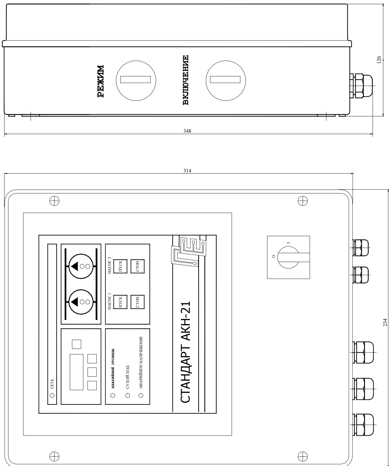
Рисунок А.1 – Общий вид устройства СТАНДАРТ АКН-21Т
